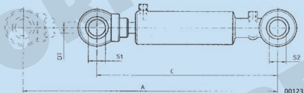
MARTINETTO CON ATTACCHI EQUIDISTANTI
